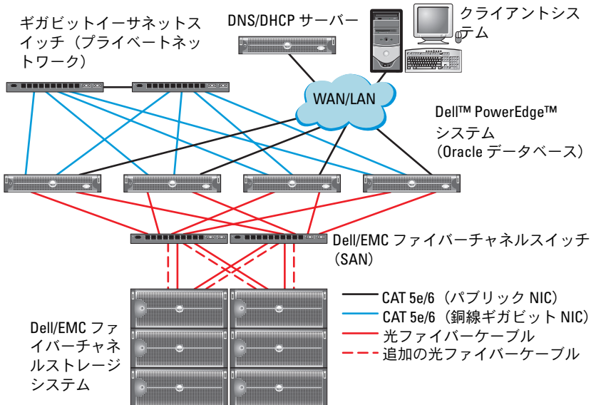
図 3-1. ファイバーチャネルクラスタ用のハードウェアの接続
